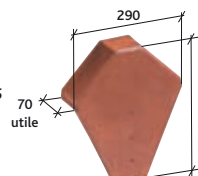
Fronton pour faîtière angulaire à emboitement Réf. 801
