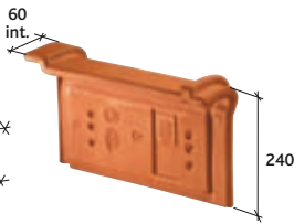
Rive universelle Réf. 1050
