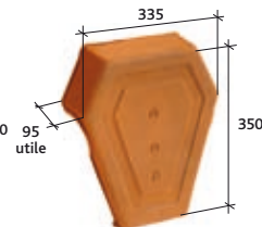
Fronton de rive universelle (1) Réf. 1080
