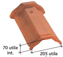
Faîtière losangée à emboitement (2,5 au ml) Réf. 716
