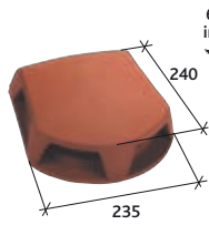
Lanterne Bi-section Ø 120 mm et 150 mm utile (Section aération 130 cm 2 ) Réf. 1000
