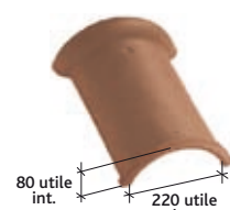
Faîtière 1/2 ronde à emboitement (2,5 au ml) Réf. 717
