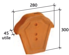
Fronton pour faîtière losangée à recouvrement Réf. 809
