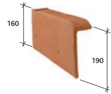
Rive individuelle gauche à emboitement Réf. 209.42
